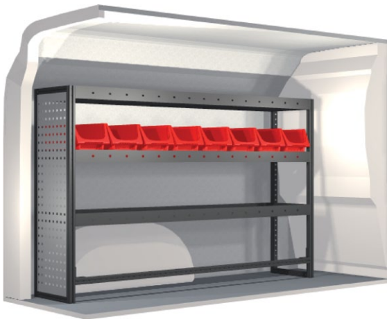
Kit n° 20100106 An. 1350 mm Pr. 324 mm Al. 918 mm Peso 28.9 kg
