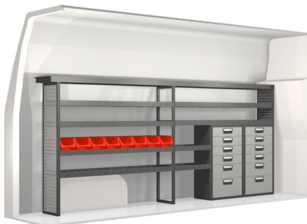
Kit n° 20100219 An. 2835 mm Pr. 324 mm Al. 1350 mm Peso 121.3 kg
