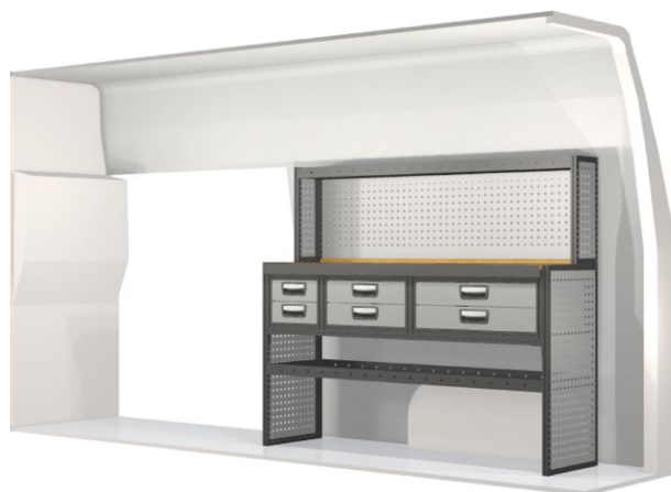
Kit n° 20100218 An. 1512 mm Pr. 486 mm Al. 1404 mm Peso 87.4 kg
