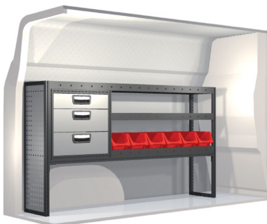
Kit n° 20100112 An. 1512 mm Pr. 324 mm Al. 918 mm Peso 41.9 kg
