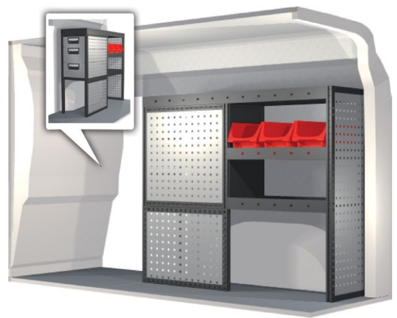
Kit n° 20100105 An. 999 mm Pr. 324 mm Al. 918 mm Peso 28.8 kg
