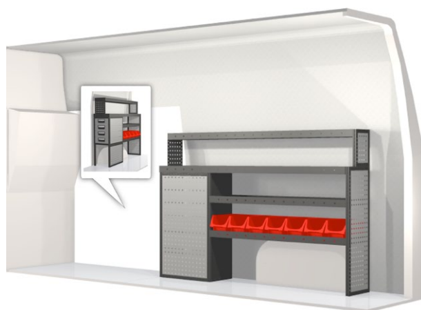
Kit n° 20100216 An. 1647 mm Pr. 324 mm Al. 1188 mm Peso 63.1 kg
