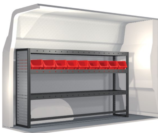
Kit n° 20100111 An. 1512 mm Pr. 324 mm Al. 918 mm Peso 37.3 kg
