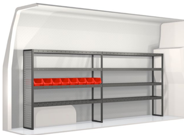
Kit n° 20100215 An. 2835 mm Pr. 324 mm Al. 1296 mm Peso 65.8 kg
