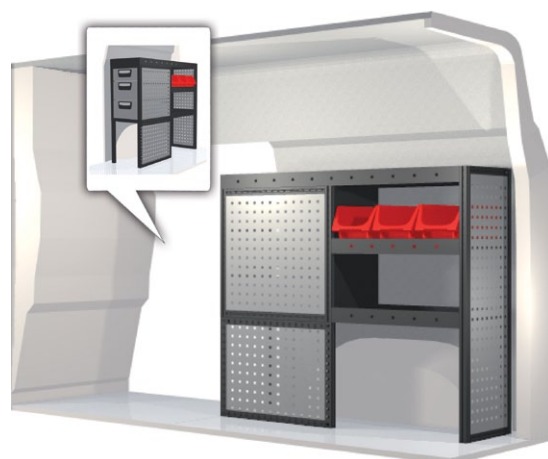
Kit n° 20100110 An. 999 mm Pr. 324 mm Al. 918 mm Peso 32.2 kg
