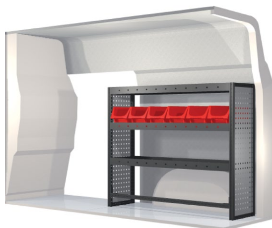
Kit n° 20100109 An. 1026 mm Pr. 324 mm Al. 918 mm Peso 24.1 kg
