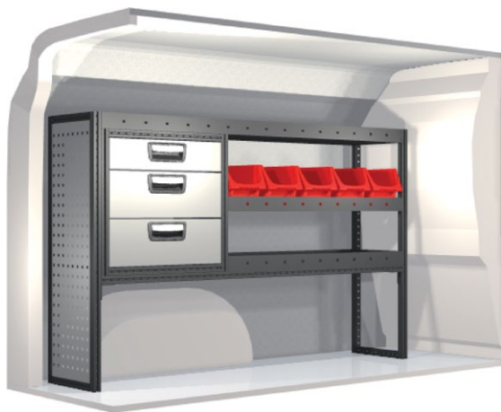
Kit n° 20100107 An. 1350 mm Pr. 324 mm Al. 918 mm Peso 39.3 kg
