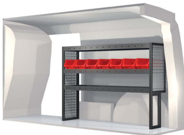
Kit n° 20100088 An. 1188 mm Pr. 324 mm Al. 918 mm Peso 25.6 kg
