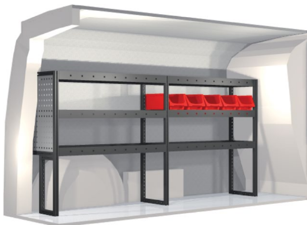
Kit n° 20100090 An. 1701 mm Pr. 324 mm Al. 918 mm Peso 32.6 kg
