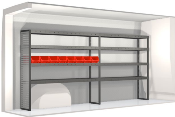
Kit n° 20100259 An. 2511 mm Pr. 324 mm Al. 1296 mm Peso 58.8 kg
