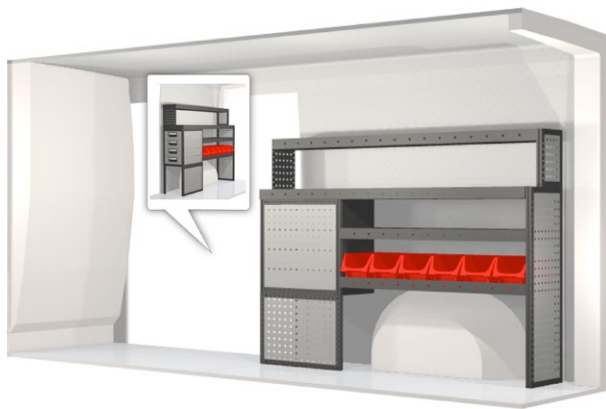
Kit n° 20100260 An. 1485 mm Pr. 324 mm Al. 1188 mm Peso 52.3 kg
