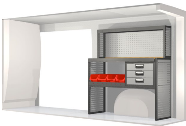
Kit n° 20100262 An. 1188 mm Pr. 486 mm Al. 1404 mm Peso 59.2 kg
