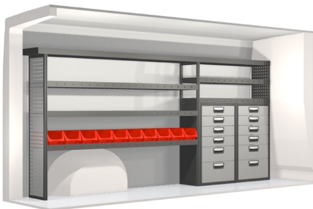
Kit n° 20100263 An. 2646 mm Pr. 324 mm Al. 1350 mm Peso 111.5 kg
