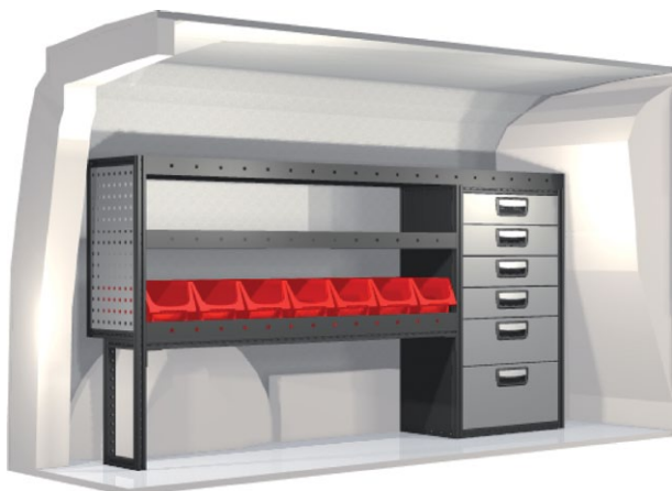
Kit n° 20100092 An. 1674 mm Pr. 324 mm Al. 918 mm Peso 53.7 kg
