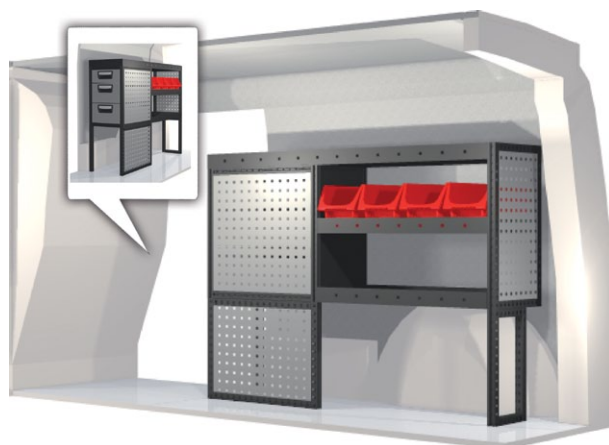
Kit n° 20100089 An. 1161 mm Pr. 324 mm Al. 918 mm Peso 35.7kg
