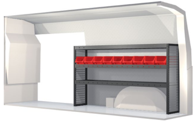
Kit n° 20100203 Pr. 1512 mm Pr. 324 mm Al. 918 mm Peso 32.4 kg
