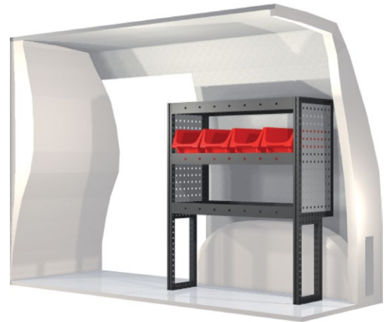
Kit n° 20100197 An. 864 mm Pr. 324 mm Al. 918 mm Peso 20.4 kg
