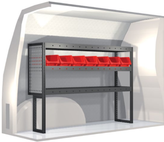
Kit n° 20100196 An. 1188 mm Pr. 324 mm Al. 918 mm Peso 24.7 kg
