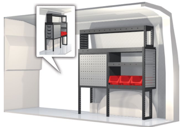
Kit n° 20100185 Pr. 999 mm Pr. 324 mm Al. 1188 mm Peso 39.7 kg
