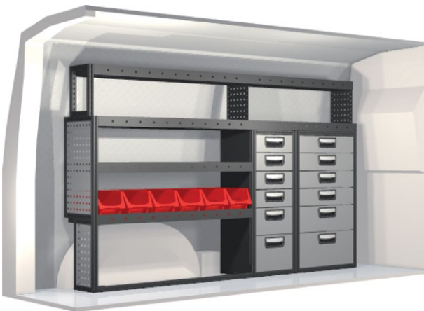
Kit n° 20100189 Pr. 1809 mm Pr. 324 mm Al. 918 mm Peso 85.5 kg
