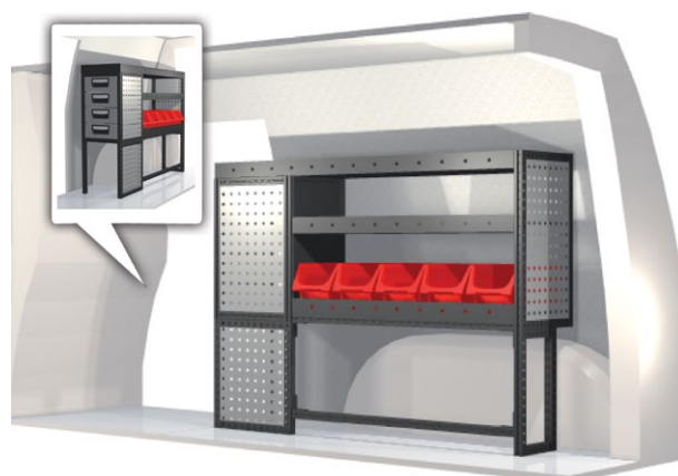
Kit n° 20100180 Pr. 1161 mm Pr. 324 mm Al. 918 mm Peso 37.9 kg
