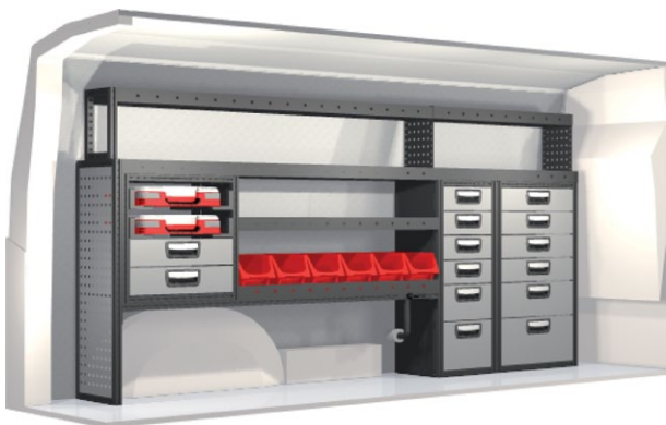
Kit n° 20100188 Pr. 2295 mm Pr. 324 mm Al. 1188 mm Peso 103.6 kg
