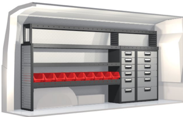
Kit n° 20100187 Pr. 2295 mm Pr. 324 mm Al. 1188 mm Peso 96 kg
