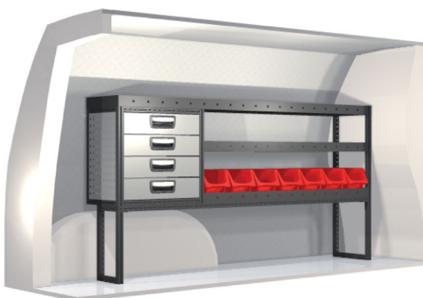
Kit n° 20100181 Pr. 1647 mm Pr. 324 mm Al. 918 mm Peso 43.6 kg
