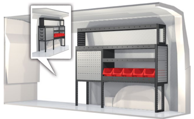
Kit n° 20100186 Pr. 1323 mm Pr. 324 mm Al. 918 mm Peso 48.8 kg
