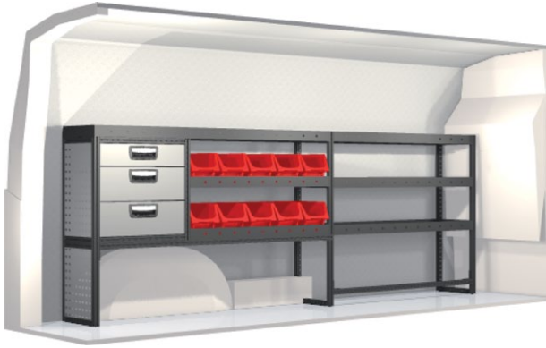
Kit n° 20100202 Pr. 2187 mm Pr. 324 mm Al. 918 mm Peso 38.9 kg
