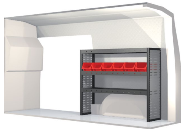
Kit n° 20100201 Pr. 1026 mm Pr. 324 mm Al. 918 mm Peso 24.4 kg
