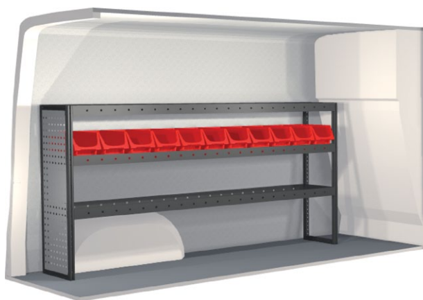
Kit n° 20100171 An. 1836 mm Pr. 324 mm Al. 918 mm Peso 40.3 kg
