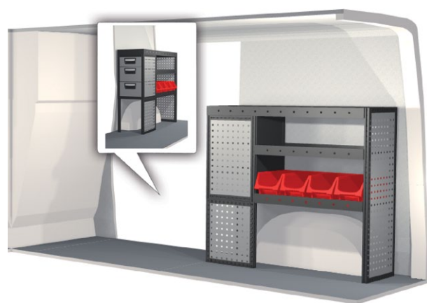
Kit n° 20100170 An. 999 mm Pr. 324 mm Al. 918 mm Peso 31.8 kg
