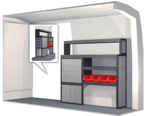
Kit n° 20100270 An. 1161 mm Pr. 324 mm Al. 1188 mm Peso 44.7 kg
