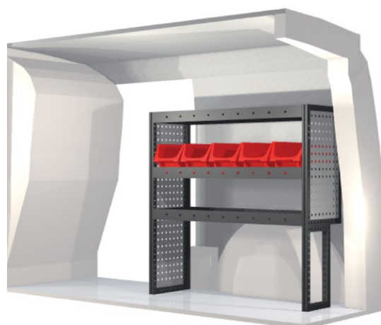
Kit n° 20100093 An. 864 mm Pr. 324 mm Al. 918 mm Peso 20.7 kg
