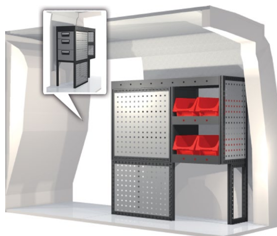
Kit n° 20100094 An. 837 mm Pr. 324 mm Al. 918 mm Peso 30.2kg
