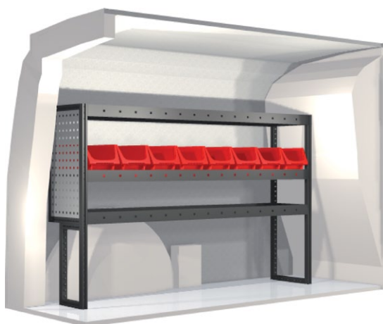
Kit n° 20100095 An. 1350 mm Pr. 324 mm Al. 918 mm Peso 28.1 kg
