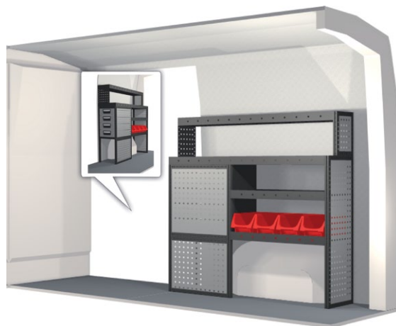
Kit n° 20100270 An. 1161 mm Pr. 324 mm Al. 1188 mm Peso 44.7 kg
