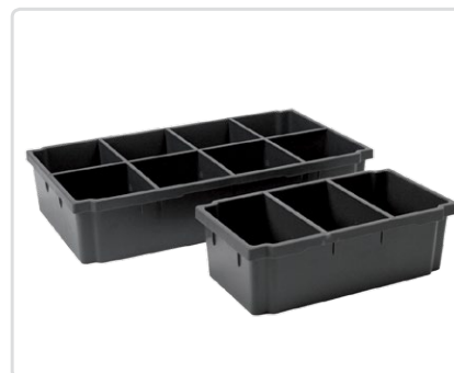
Insertos para cajones For 108 mm cajón alto, Ref. n° 10530-03* For 108 mm cajón alto, Ref. n° 10533-03** For 162/216 mm cajón alto, Ref. n° 10535-03*** *162 mm Longitud, 324 mm Pr., **324 mm Longitud, 486 mm Pr., ***324 mm Longitud, 324 mm Pr.
