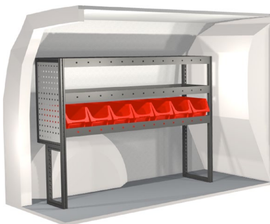
Kit n° 20100166 An. 1188 mm Pr. 324 mm Al. 918 mm Peso 24.1 kg
